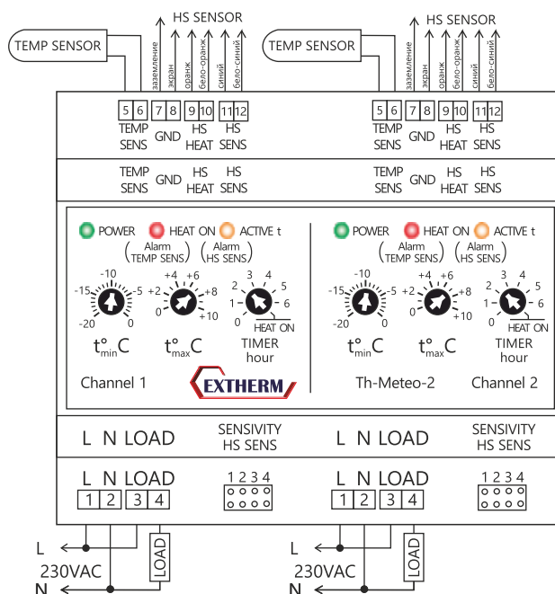
Схема подключения
