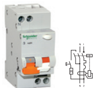
Дифференциальный автоматический выключатель
